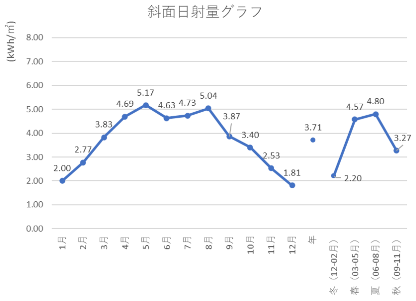
図 3:北栄町由良駅付近の月・年・季節平均の日射量(kWh/m 2 ・day)、水平から傾斜角 30 度、方位角 45 度(南西)に向けた太陽光発電のパネル 1 m 2 に降り注ぐ 1 日あたりの日射量(出典: NEDO、年間月別日射量データベース https://appww2.infoc.nedo.go.jp/appww/monsola.html?m=53331680 )
