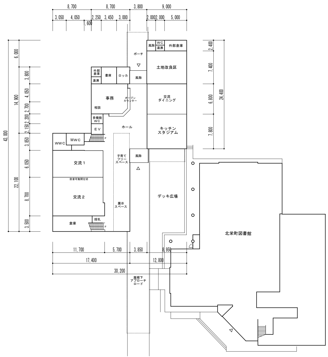
1階 平面図
